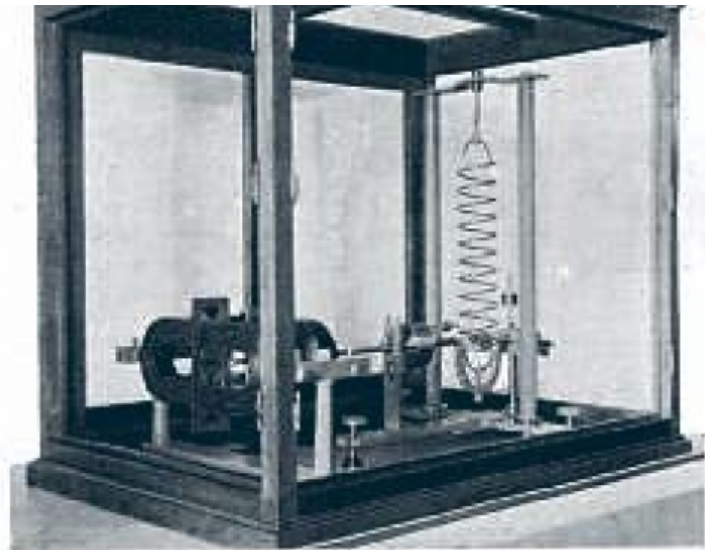
Componente vertical «Belarmino» de la Estación de Cartoja (Granada)
